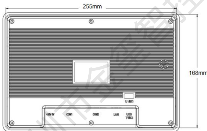
背面
