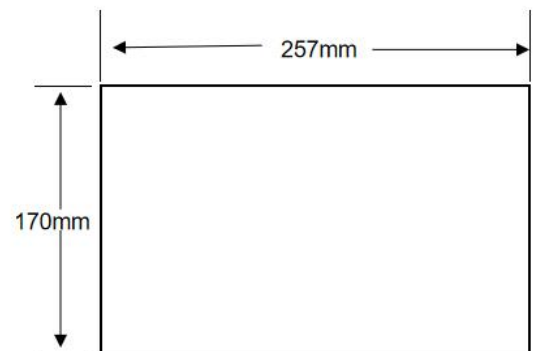
建议开孔尺寸
